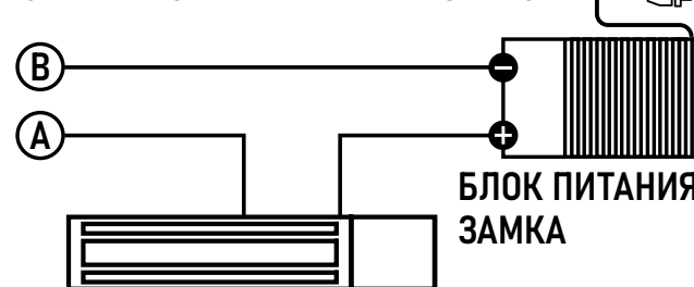
Рис. 6 Стандартная схема подключения вызывной панели
