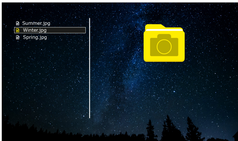
Рис. 3014 Просмотр фото
