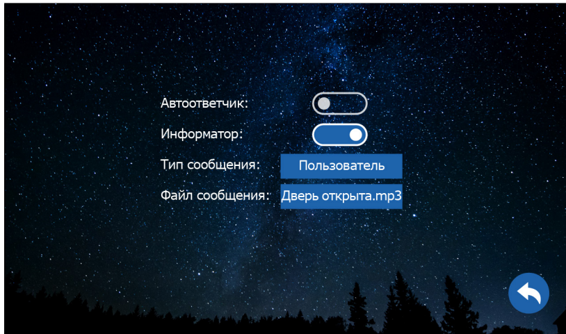
Рис. 23 Подменю "Сообщения"
