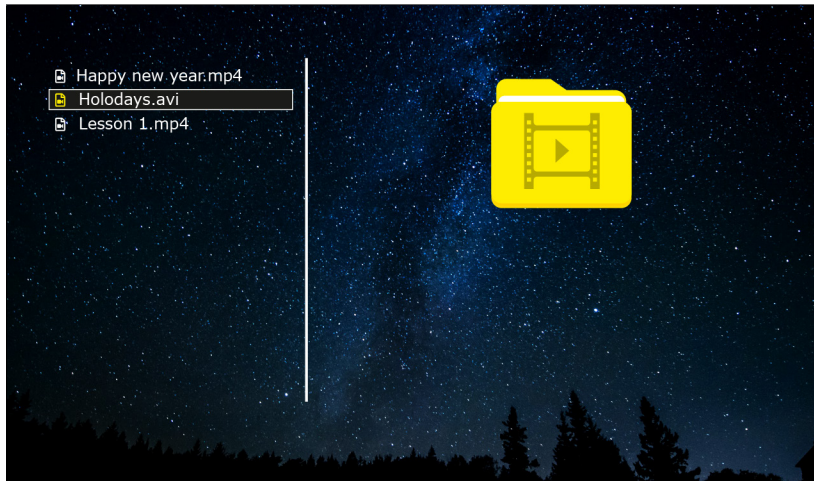
Рис. 29 Проигрывание видео
