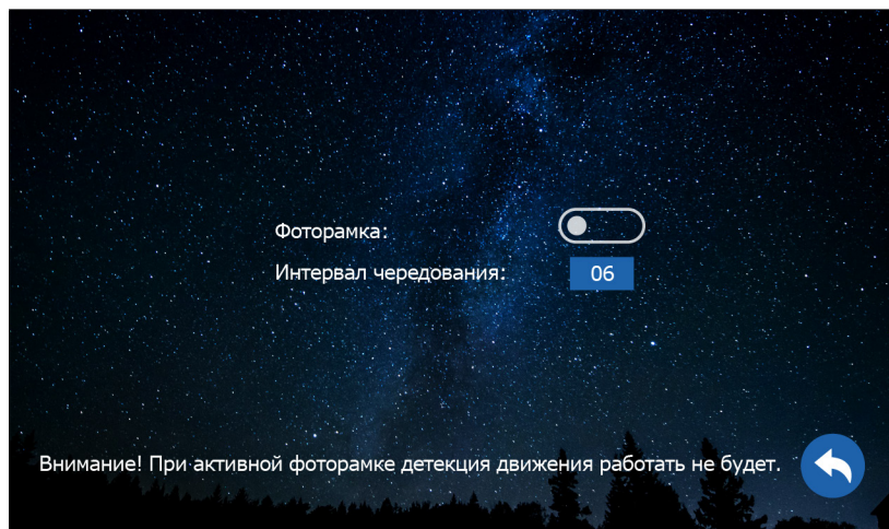
Рис. 24 Подменю "Фоторамка"
