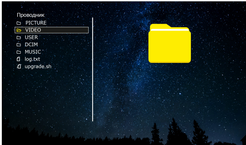
Рис. 31 Проводник
