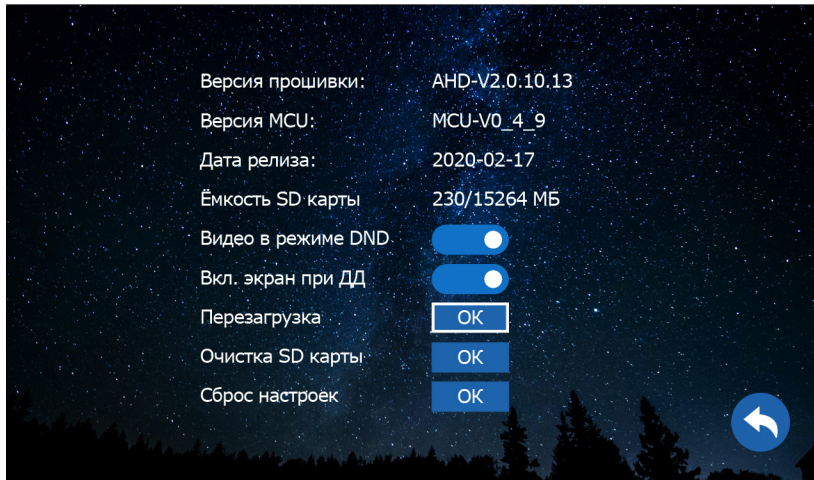
Рис. 25 Подменю "Управление"
