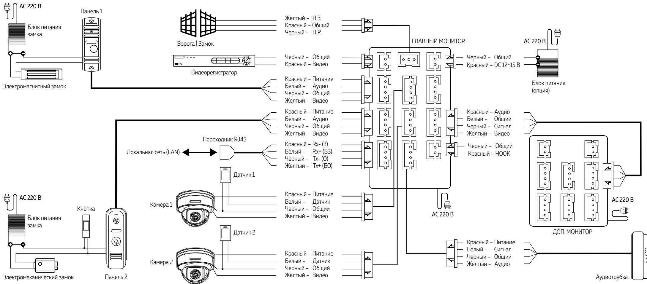
Рис. 9 Схема подключения видеодомофонов FREEDOM FHD WIFI
